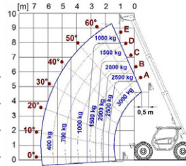
Ulottuma ilman tukijalkoja
