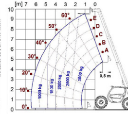
Ulottuma tukijalat maassa
